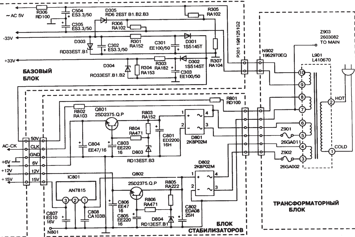
Принципиальная схема источника питания видеомagniтофона SV-T25 фирмы SUPRA.
